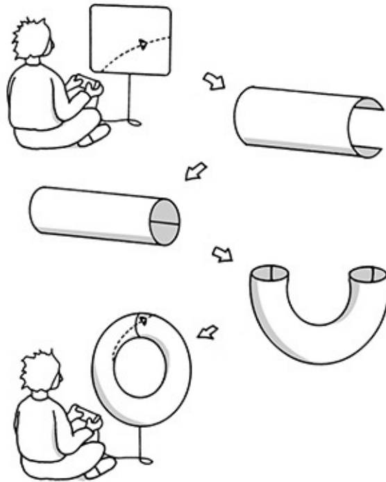
Figura 9.2. Se um foguete desaparece pelo lado direito de uma tela de videogame, ele ressurgirá à esquerda. Se desaparece no alto, reaparece embaixo. Vamos agora enrolar a tela de modo que pontos idênticos se encontrem. Primeiro fazemos encontrar as pontas de cima e a de baixo enrolando a tela. Depois, fazemos coincidir os pontos da esquerda e da direita encurvando a tela como um tubo. Dessa maneira, podemos mostrar que a tela de um videogame tem a topologia de uma rosca.
