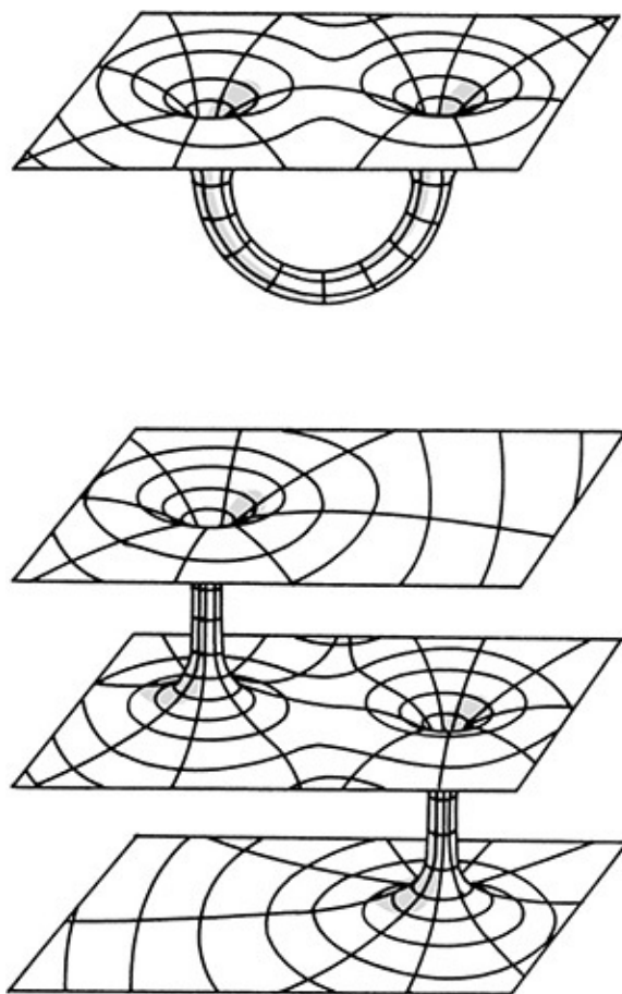
Figura 1.2. Buracos de minhoca podem conectar um universo consigo mesmo, tornando possível uma viagem interestelar. Assim como podem conectar duas eras diferentes, os buracos de minhoca podem também conectar uma série infinita de universos paralelos. A esperança é que a teoria do hiperespaço venha a ser capaz de determinar se os buracos de minhoca são fisicamente possíveis ou uma mera curiosidade matemática.
