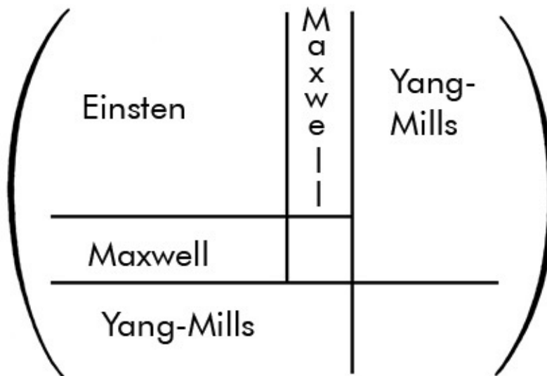
Figura 6.2. Se vamos à enésima dimensão, então o tensor métrico é uma série de N^2 números que podem ser arranjados num bloco N \times N . Removendo as quintas e mais altas colunas e fileiras, podemos extrair o campo eletro magnético de Maxwell e o campo de Yang-Mills. Assim, de um só golpe, a teoria do hiperespaço nos permite unificar o campo de Einstein (que descreve a gravidade), o campo de Maxwell (que descreve a força eletromagnética) e o campo de Yang-Mills (que descreve a força fraca e a forte). As forças fundamentais se encaixam exatamente como as peças de um quebra-cabeça.
