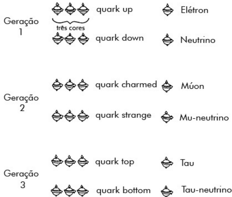
Figura 5.4. No Modelo Padrão, a primeira geração de partículas consiste nos quarks “up” e “down” (em três cores, com suas antipartículas associadas) e o elétron e o neutrino. A característica embaraçosa do Modelo Padrão é que há três gerações de tais partículas, cada uma sendo quase a cópia exata da geração anterior. É difícil acreditar que a natureza seria redundante a ponto de criar, num nível fundamental, três cópias idênticas de partículas.
