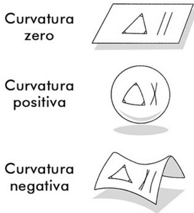
Figura 2.2. Um plano tem curvatura zero. Na geometria euclidiana, os ângulos internos de um triângulo somam 180 graus e linhas paralelas nunca se encontram. Na geometria não euclidiana, uma esfera tem curvatura positiva. Os ângulos internos de um triângulo somam mais de 180 graus e linhas paralelas sempre se encontram. (As linhas paralelas incluem arcos cujos centros coincidem com o centro da esfera. Isso exclui linhas latitudinais.) Uma sela tem curvatura negativa. Os ângulos internos somam menos de 180 graus. Há um número infinito de linhas paralelas a uma dada linha que atravessam um ponto fixo.
