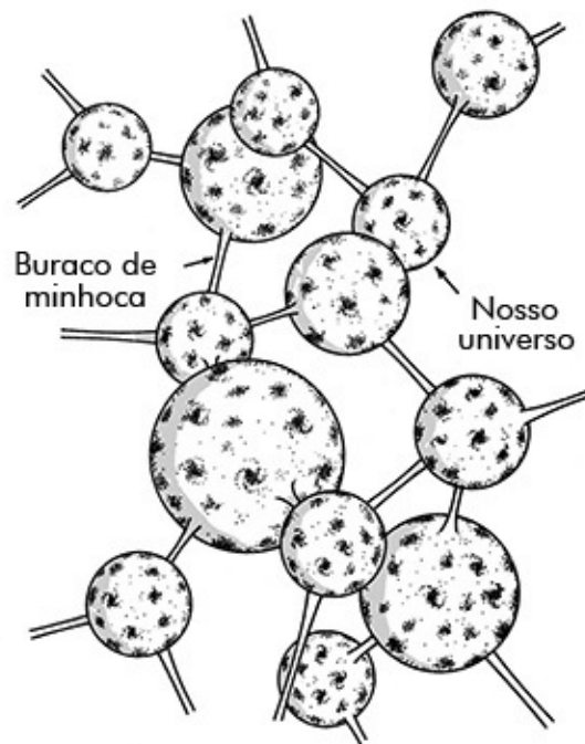
Figura 12.2. Nosso universo pode ser um de um número infinito de universos paralelos, cada um ligado aos demais por uma série infinita de buracos de minhoca. Viajar entre esses buracos de minhoca é possível mas extremamente improvável.
