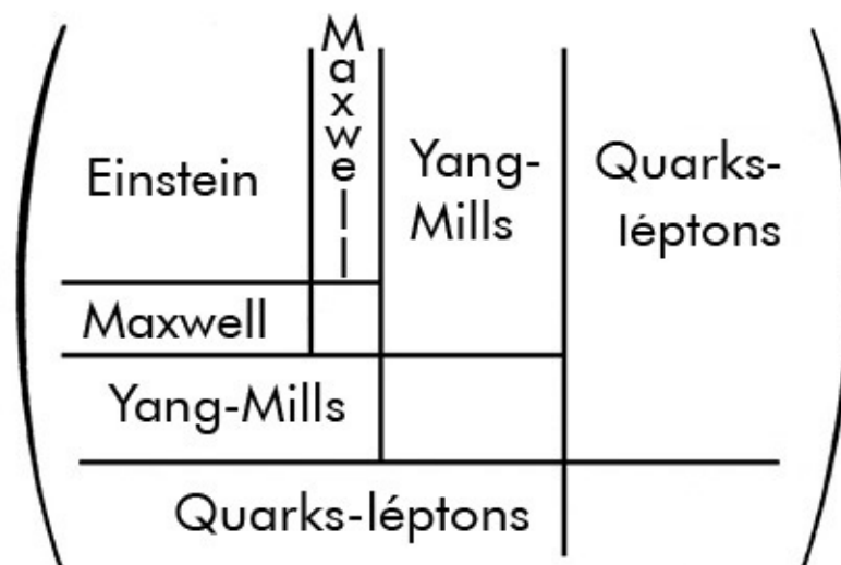
Figura 6.3. A super gravida de quase realiza o sonho de Einstein de dar uma derivação puramente geométrica de todas as forças e partículas no universo. Para ver isso, note que se acrescentarmos supersimetria ao tensor métrico de Riemann, a métrica dobra em tamanho, dando-nos a supermétrica de Riemann. Os novos componentes do supertensor de Riemann correspondem a quarks e léptons. Mas se fatiarmos o supertensor de Riemann em seus componentes, verificamos que ele inclui quase todas as partículas e forças fundamentais da natureza: a teoria da gravidade de
