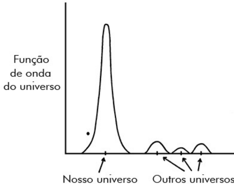
Figura 12.1. Na função de onda do universo de Hawking, a função de onda está provavelmente mais concentrada em torno do nosso universo. Vivemos no nosso universo porque ele é o mais provável, tem a maior probabilidade. No entanto, há uma pequena mas não evanescente probabilidade de que a função de onda prefira universos vizinhos, paralelos. Portanto, transições entre universos podem ser possíveis (embora com probabilidade muito baixa).
