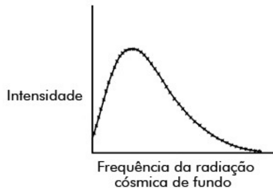
Figura 9.1. A linha sólida representa a previsão feita pela teoria do Big Bang, segundo a qual a radiação cósmica de fundo deveria se assemelhar à radiação do corpo negro na região das micro-ondas. Os x representam os dados reais coletados pelo satélite COBE, fornecendo-nos uma das mais convincentes provas da teoria do Big Bang.
