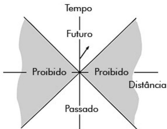
Figura 11.1. Nossa linha de mundo sintetiza toda a nossa história, do nascimento à morte. Por exemplo, se ficamos na cama das 08:00 às 12:00h, nossa linha de mundo é uma linha vertical. Se vamos de carro para o trabalho, nossa linha de mundo se torna uma linha inclinada. Quanto mais depressa nos movermos, mais inclinada se torna nossa linha de mundo. A rapidez máxima com que podemos nos mover, no entanto, é a velocidade da luz. Assim, parte do diagrama de espaço-tempo é “proibida”; isto é, teríamos de nos mover numa velocidade maior que a da luz para entrar nessa zona proibida.
