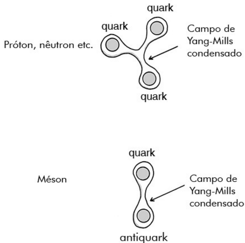
Figura 5.3. As partículas de interação forte são na realidade compósitos de partículas ainda menores, chamadas quarks, que são ligadas por uma “cola” semelhante a uma goma, que é
