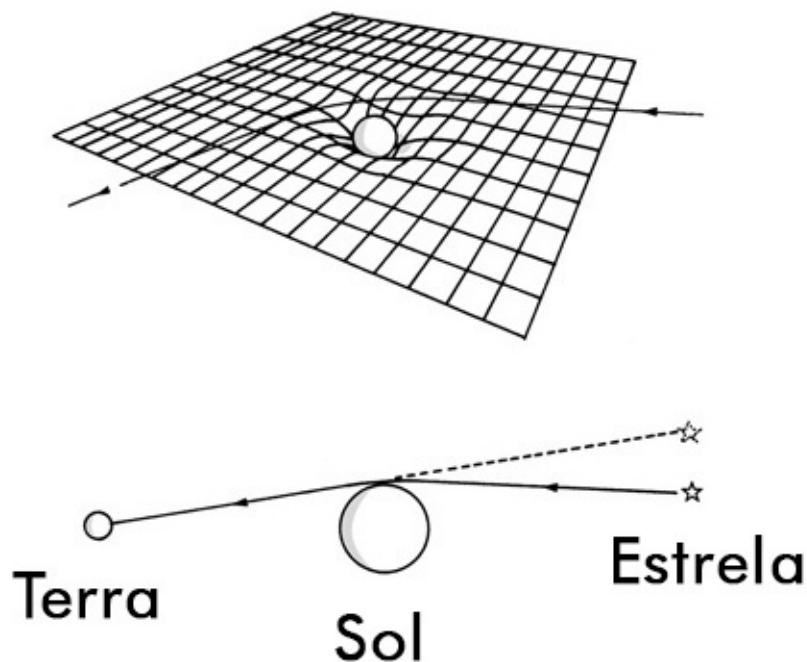
Figura 4.1. Para Einstein, a “gravidade” era uma ilusão causada pelo encurvamento do espaço. Ele previu que a luz das estrelas, ao se mover em torno do Sol, seria curvada, e por isso as posições relativas das estrelas deveriam aparecer distorcidas na presença do Sol. Isso foi verificado por repetidos experimentos.
