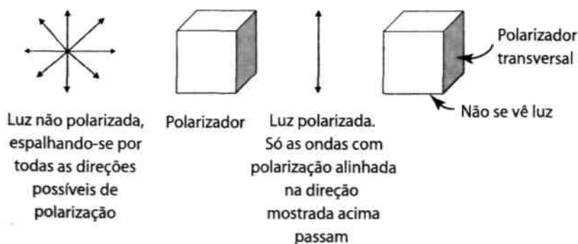
Figura 2.8 O aspecto duplo da polarização é revelado quando se observa a luz por polaroids cruzados: não se enxerga nada.
